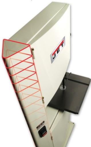
Delta-design av maskinkropp for optimal stabilitet og styrke
