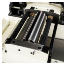
Kutterblokk og matevalser
