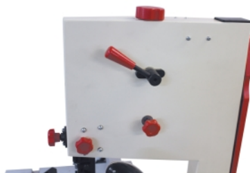
Hurtigutløser for bladstamming
